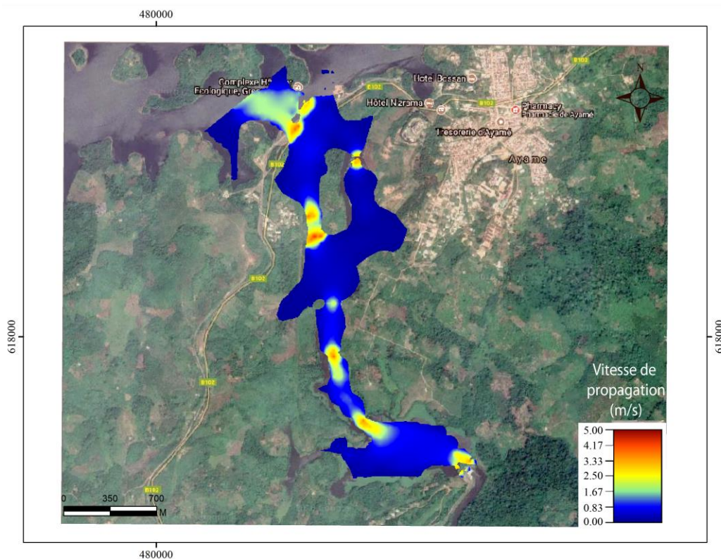
Figure 40 : Inondation prévue 1 mn 42 s après la rupture du barrage d'Ayamé 1
