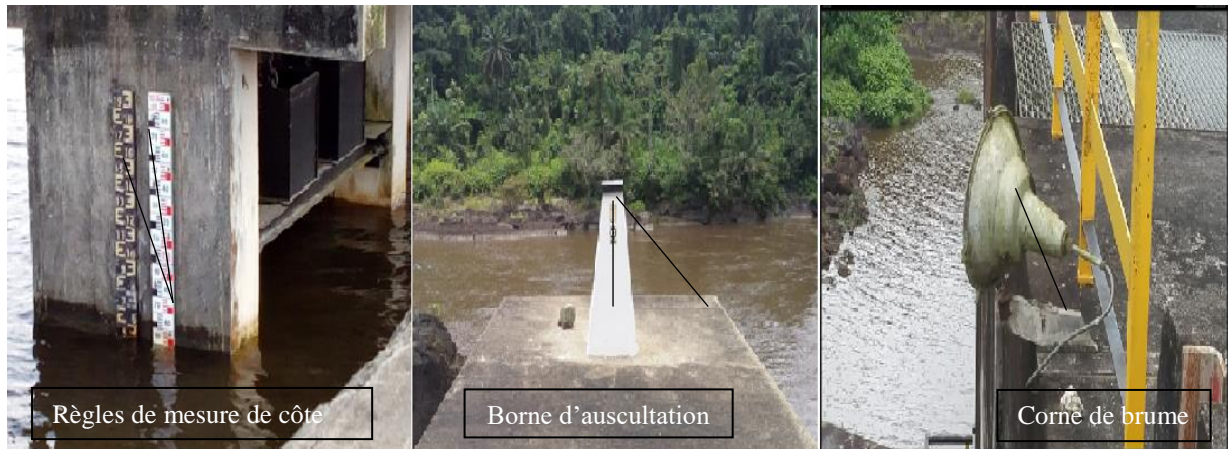
Planche 5 : Outils de sécurité des barrages d'Ayamé
